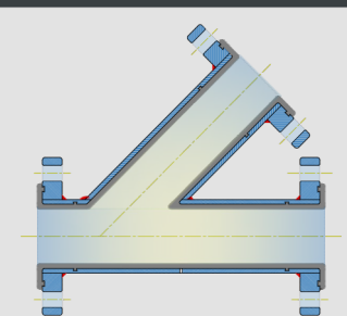
LATERAL TEE
